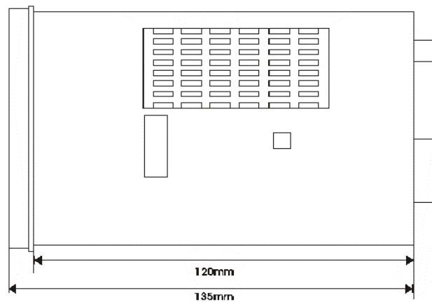
侧视图 外形结构图
