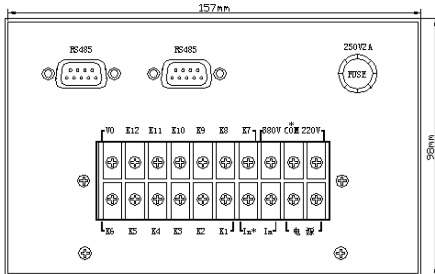
背板接线图
