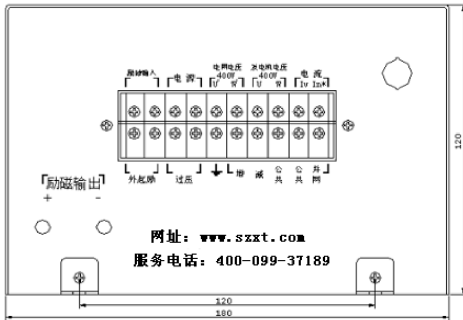
背面接线图
